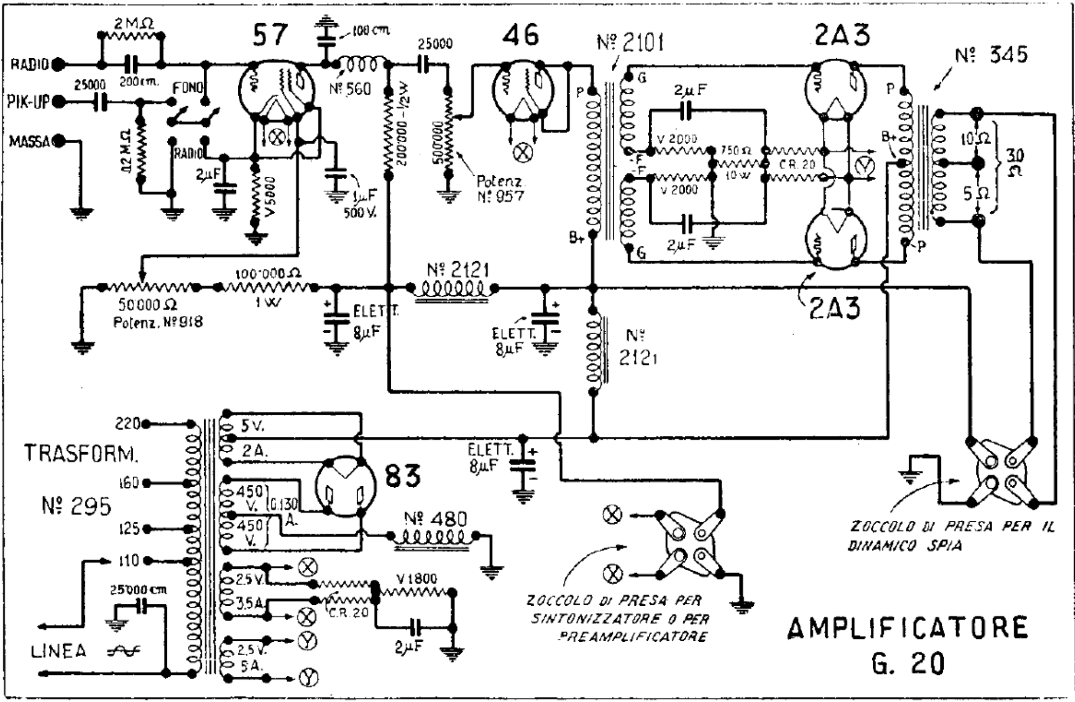
Lo schema elettrico dell'amplificatore G-20.
